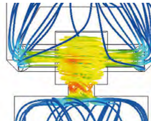
Schematische Darstellung der Micro-Levitation: (Wassereintritt von oben)
